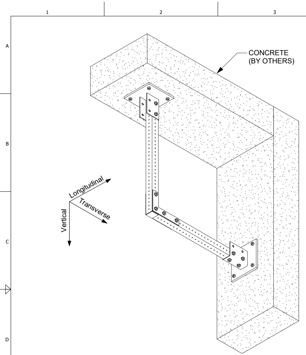
1 ISOMETRIC N.T.S.
