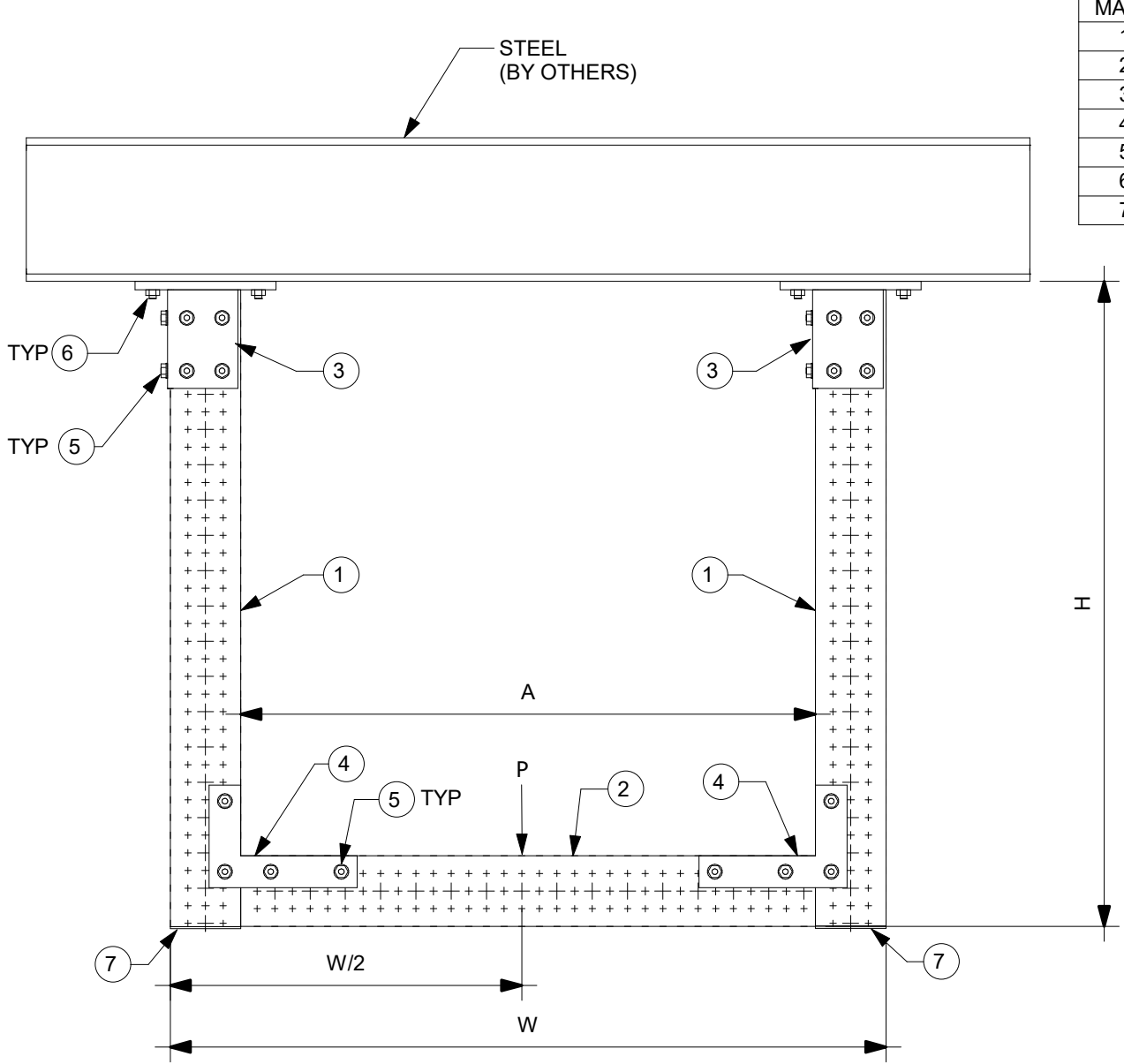
2 ELEVATION N.T.S.
