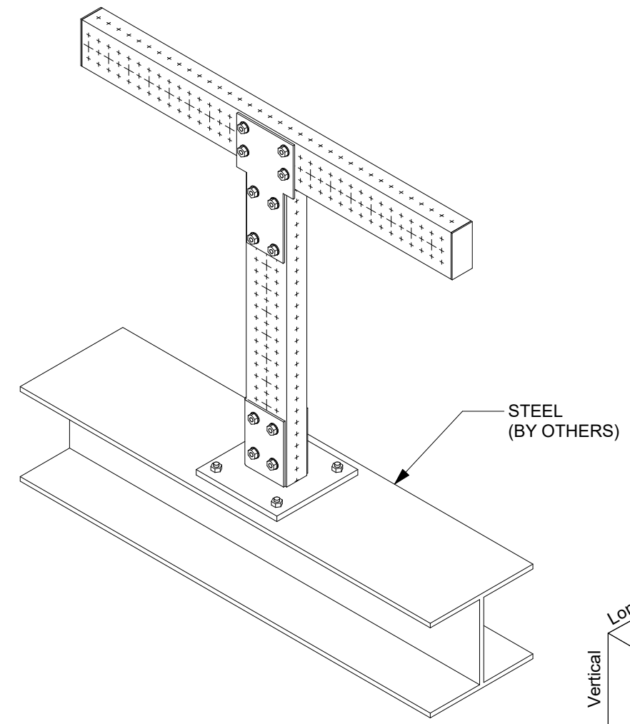
1 ISOMETRIC N.T.S.
