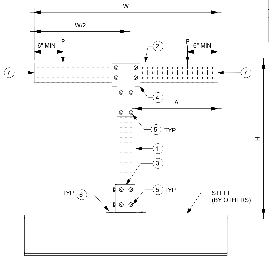
2 ELEVATION N.T.S.
