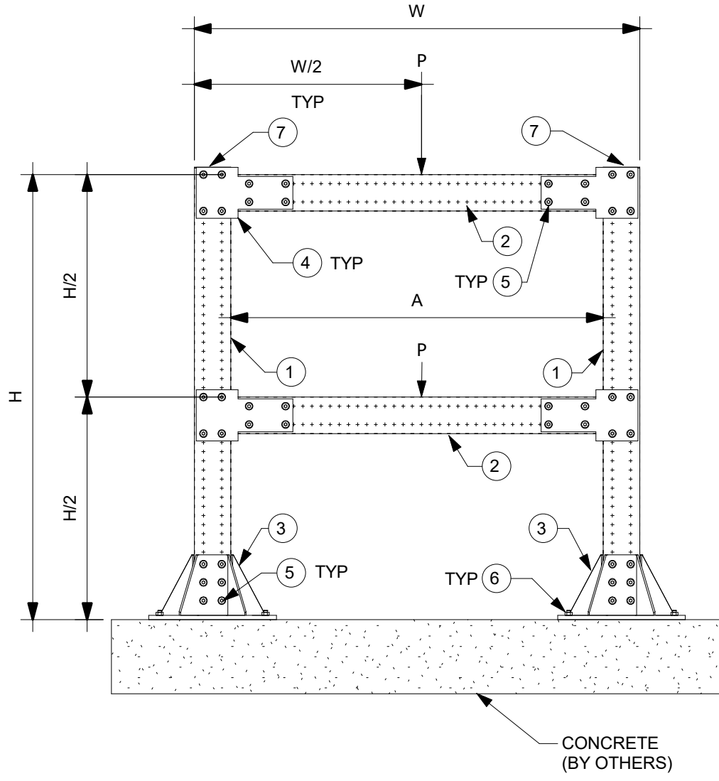
2 ELEVATION N.T.S.
