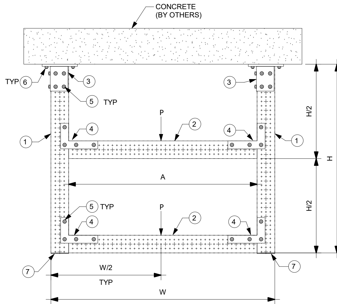
2 ELEVATION N.T.S.
