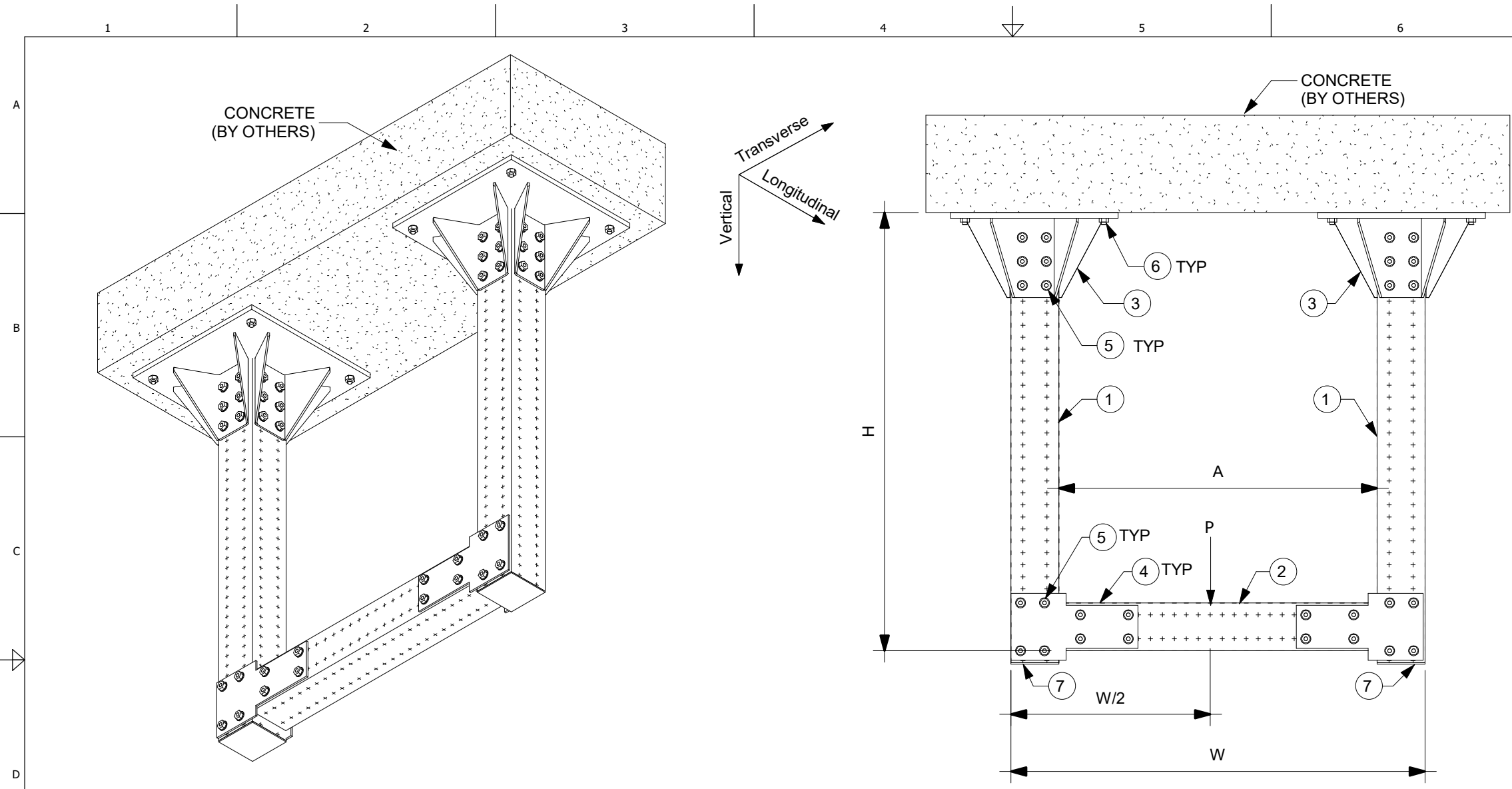
1 ISOMETRIC N.T.S.
