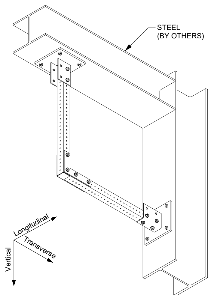
1 ISOMETRIC N.T.S.
