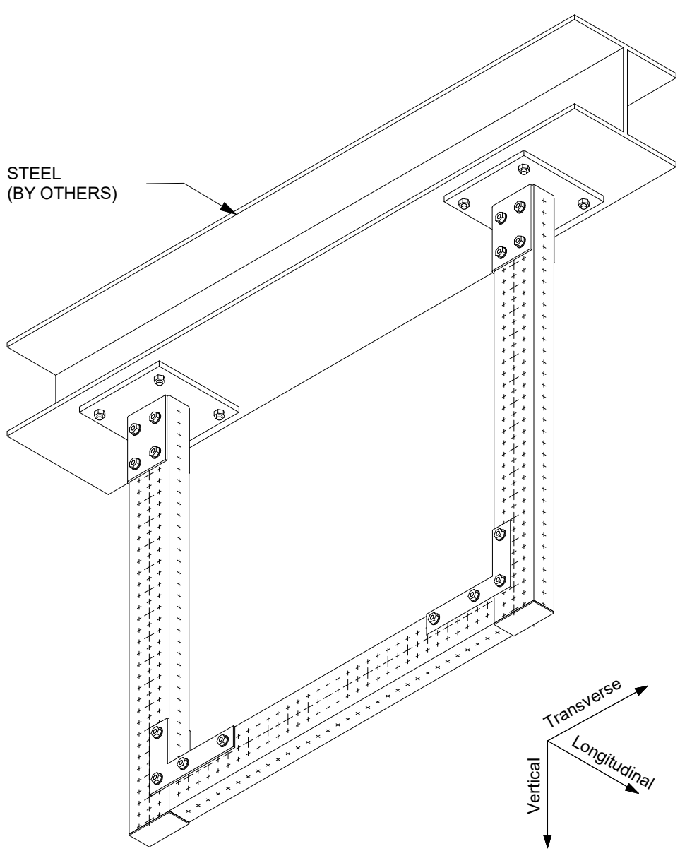
1 ISOMETRIC N.T.S.
