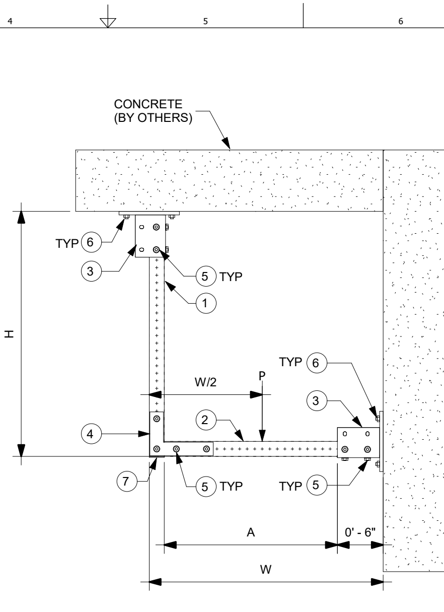
2 ELEVATION N.T.S.
