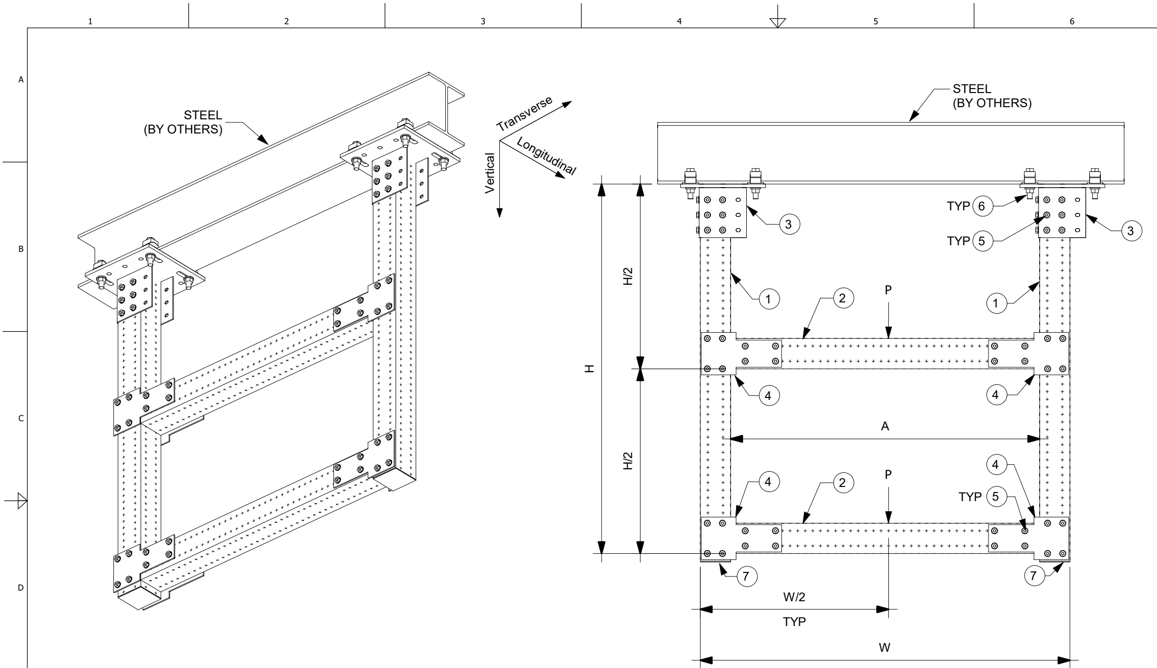
1 ISOMETRIC N.T.S.
